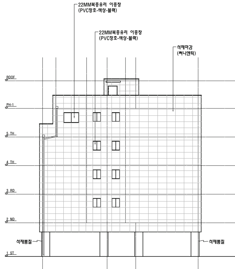
서측 면도
