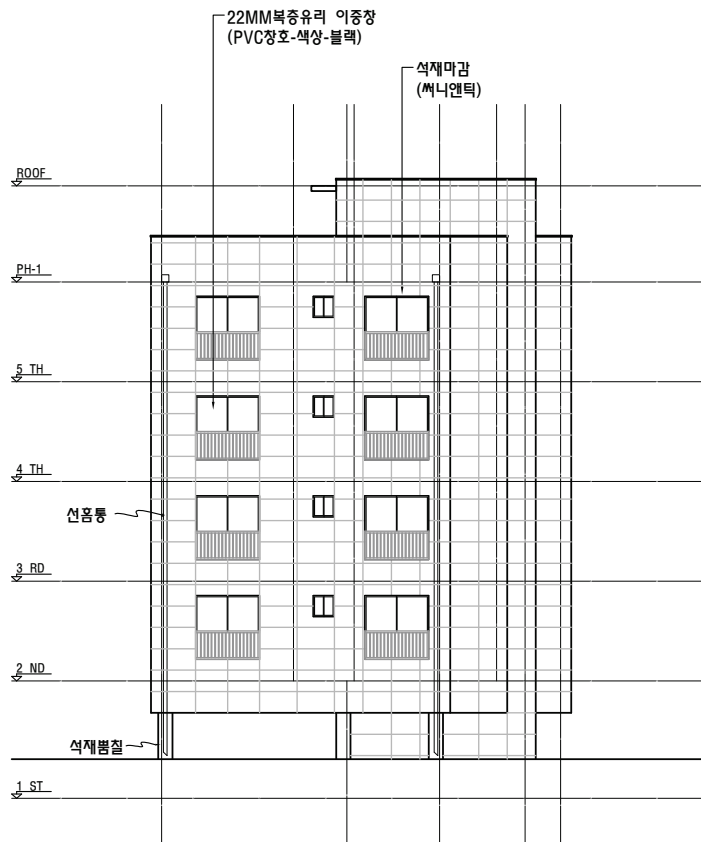
남측 면도
