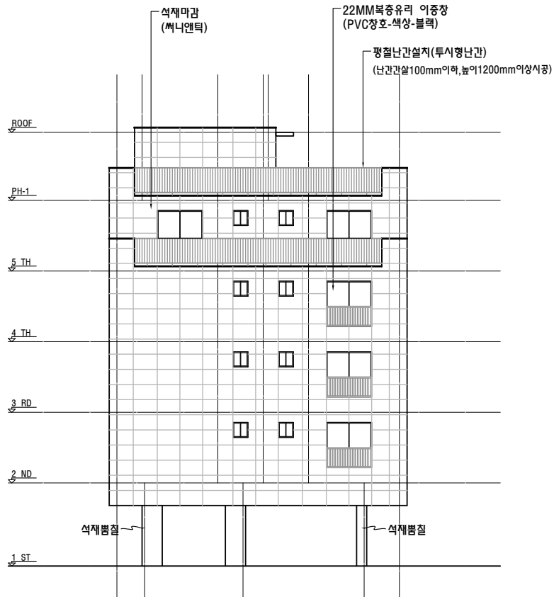
북측 면도
