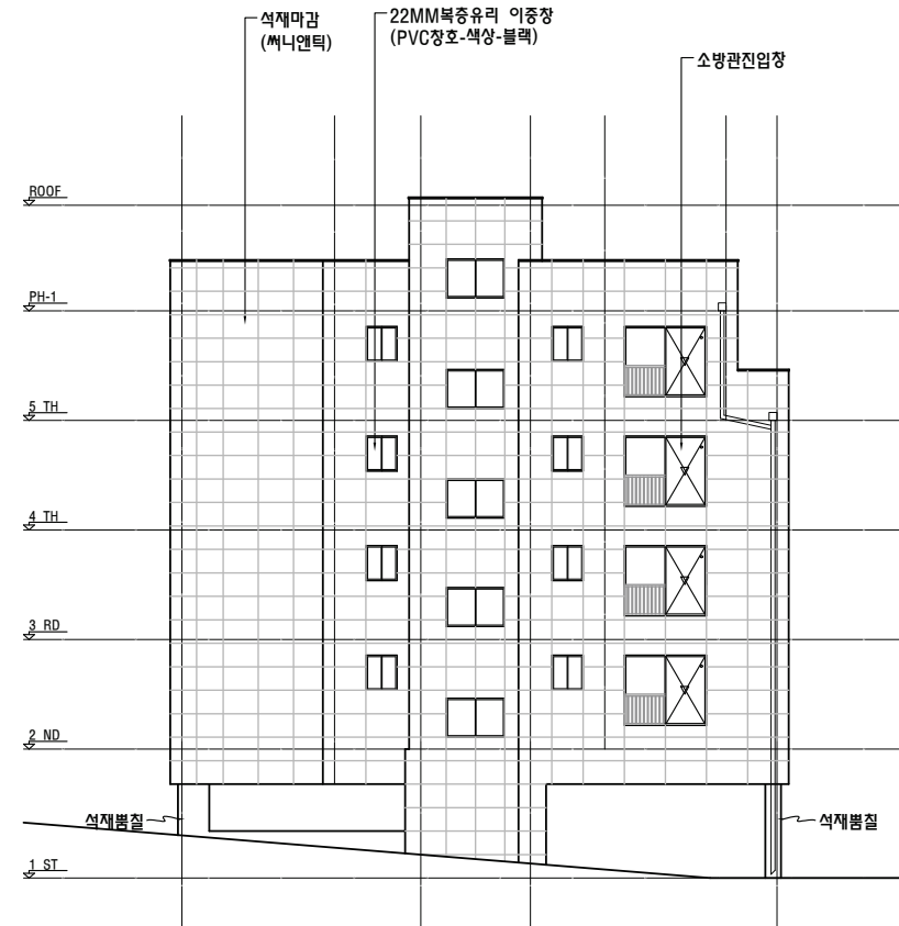
동측 면도
